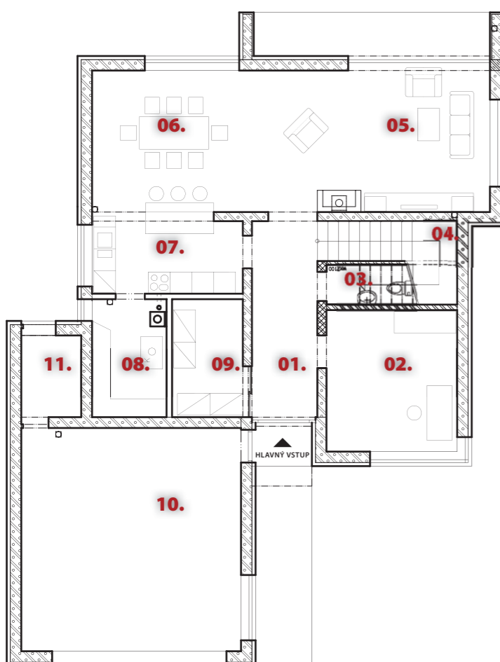
PÔDORYS PRÍZEMIA/FIRST FLOOR
